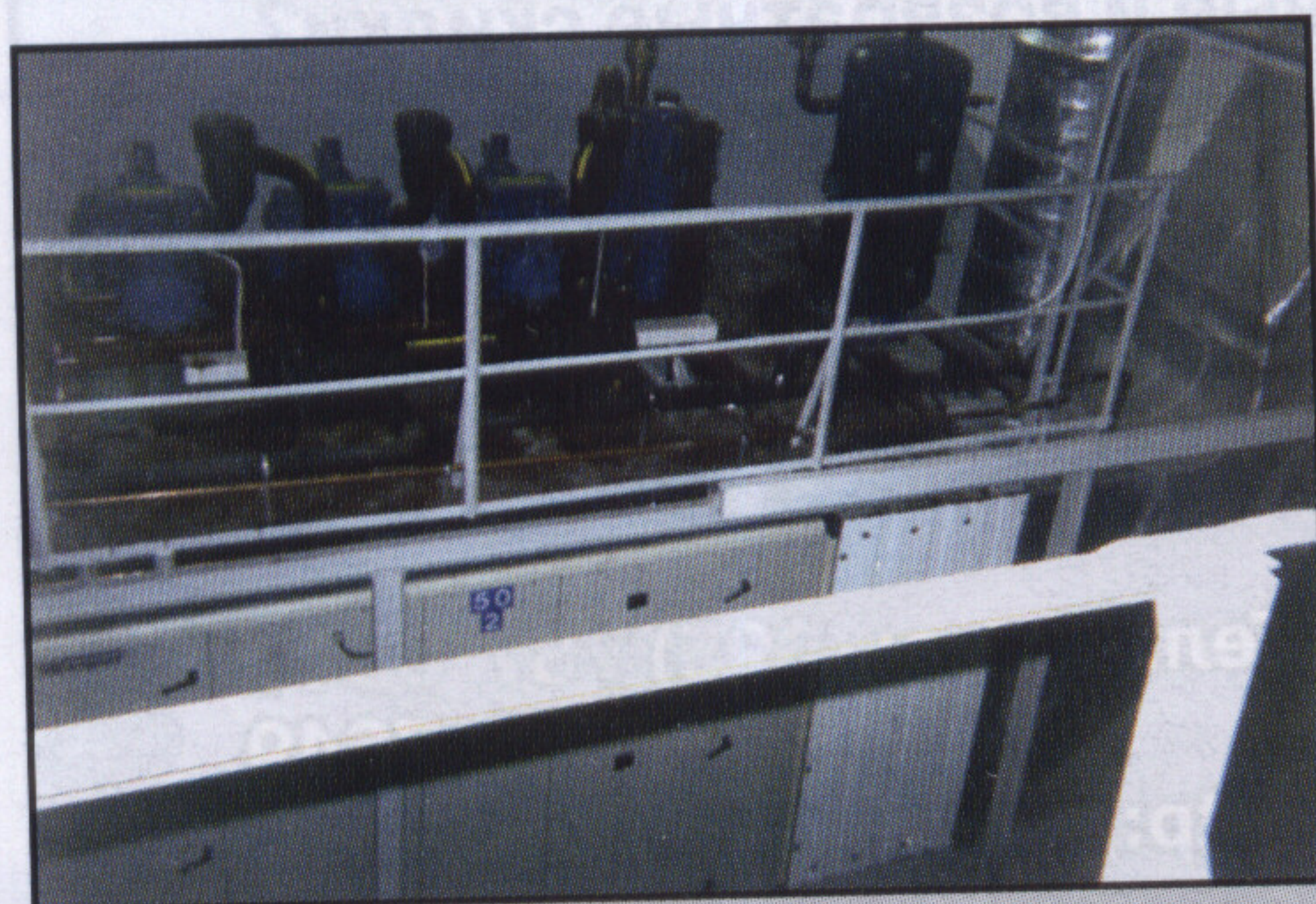
Двухъярусная конструкция с приточно-вытяжной установкой Wesper в нижнем ярусе и холодильной установкой ТЕКО в верхнем
