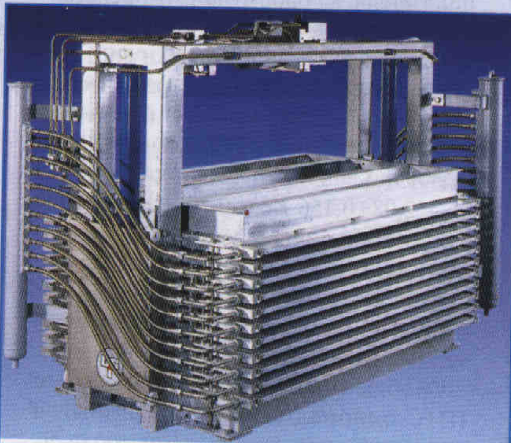
Горизонтальный плиточный скороморозильный аппарат DSI
