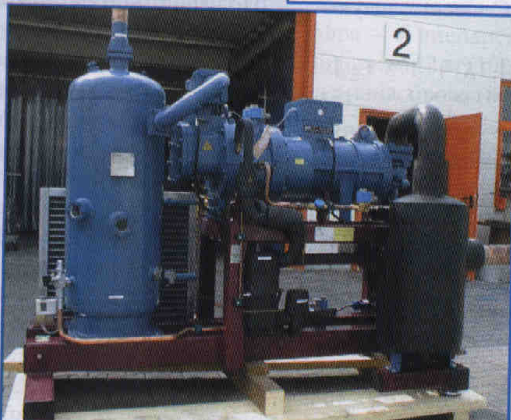
Агрегат ТЕКО на базе винтового компрессора FRASCOLD
