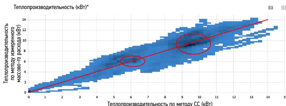
Рис. 8. Сравнение теплопроизводительность по методу CC с измеренным массовым расходом. Fig. 8. Comparison of Heating Capacity using CC method with Measured Mass Flow.
