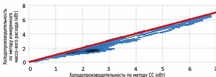
Рис. 10. Сравнение холодопроизводительности по методу СС с измеренным массовым расходом.
