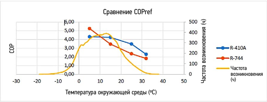
Рис. 2. Сравнение параметров R744 и R410A в зависимости от температуры в бункере и частоты возникновения. Fig. 2. COPref comparison between R-744 and R-410A based on bin temperatures and occurrences.
